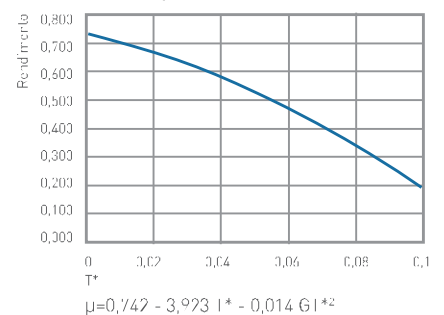
Curvas de rendimento SLIM 250
