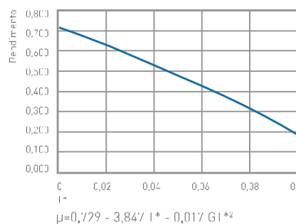
Curvas de rendimento SLIM 200
